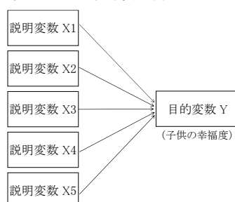
図表 5-1. 重回帰分析のイメージ
